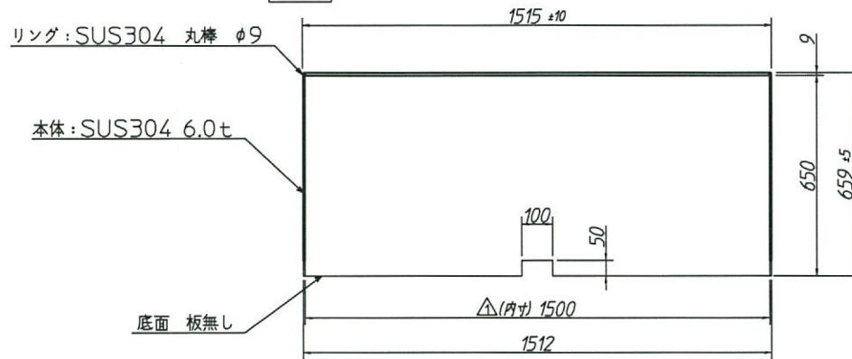
断面図
