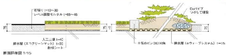
断面詳細図 1/15
